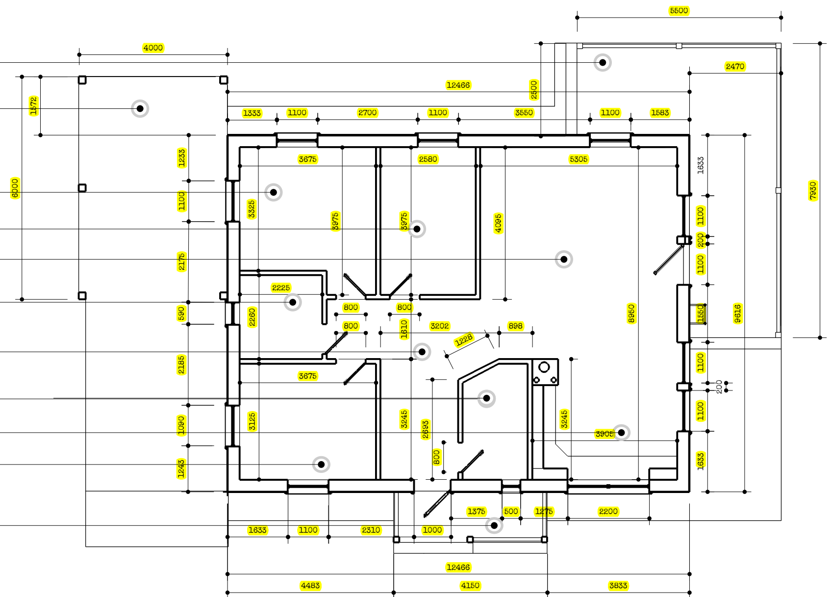
Plan M 1:100
